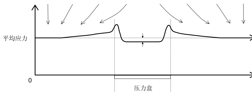
图 3 - 应力重新分布，硬土对柔性土压计
