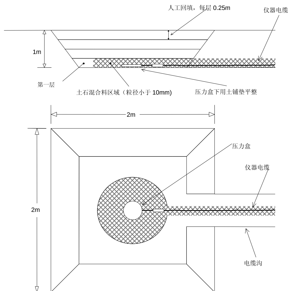
图 8 - 4800 型土压力计安装
