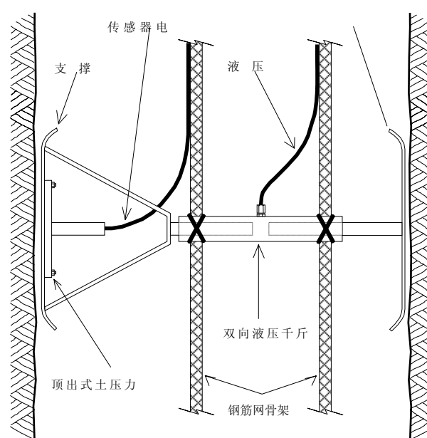
图 11 - 4820 型顶出式压力计安装
