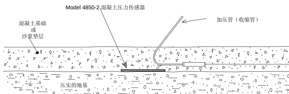
图 12 - 4850-2 型混凝土应力计安装
