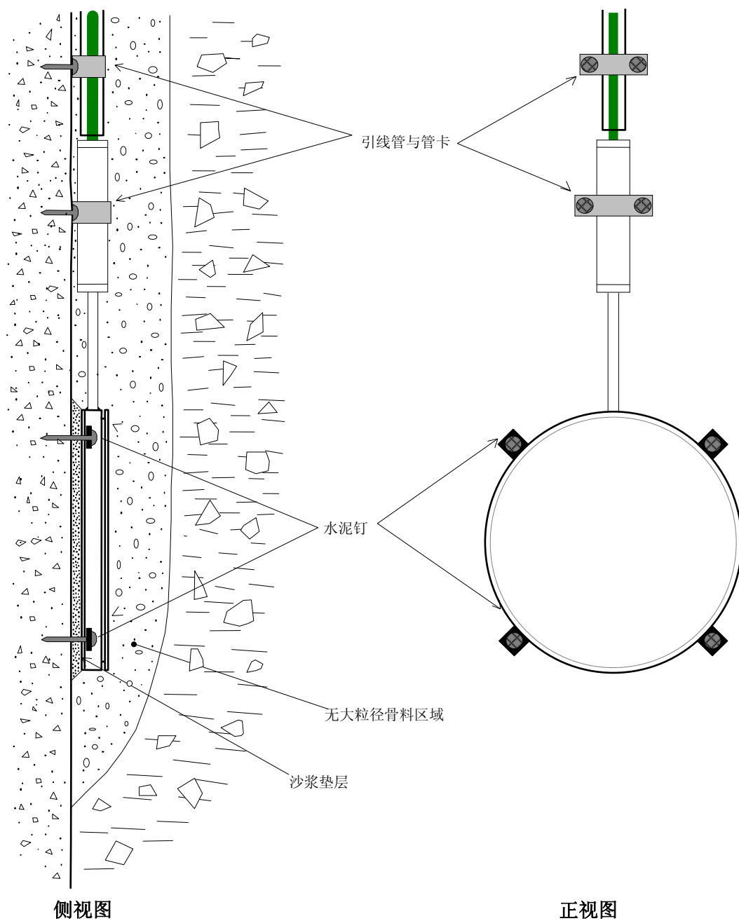
图 10 4810 型接触式土压力计安装
