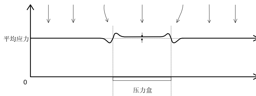
图 1 - 应力重新分布，软土用刚性土压计
