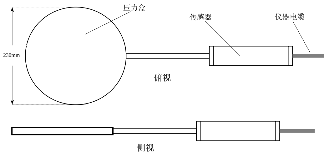
图 5 - 4800 型圆形土压力计
