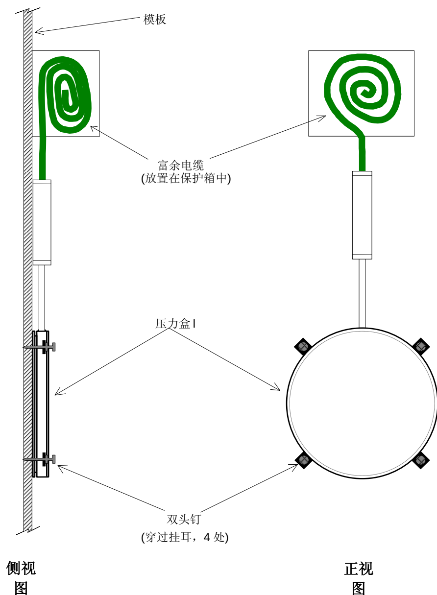
图 9 - 4810 型在模板上的固定
