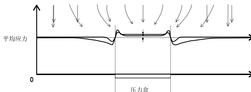
图 2 - 应力重新分布，硬土用刚性土压计
