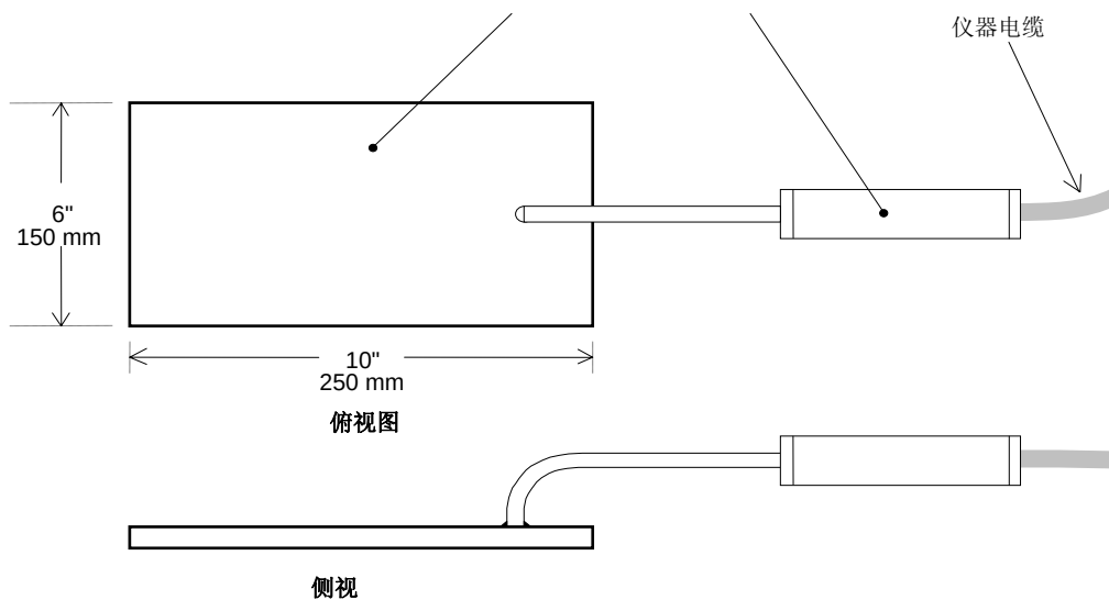
图 4 - 4800 型矩形土压力计
